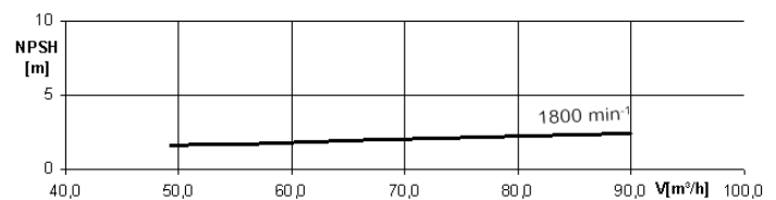
Kennlinie Wasserpumpe
