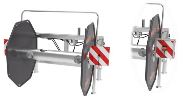
Schlauchhaspel mit optionaler Beleuchtungseinrichtung. Die steckbare Ausführung ermöglicht sowohl den Front- als auch den Heckanbau.
